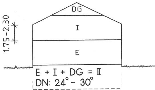
SCHEMASCHNITTE M 1/250
